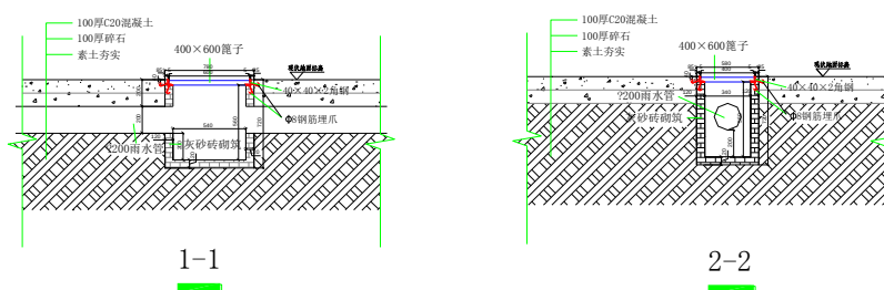
室外排水沟做法
