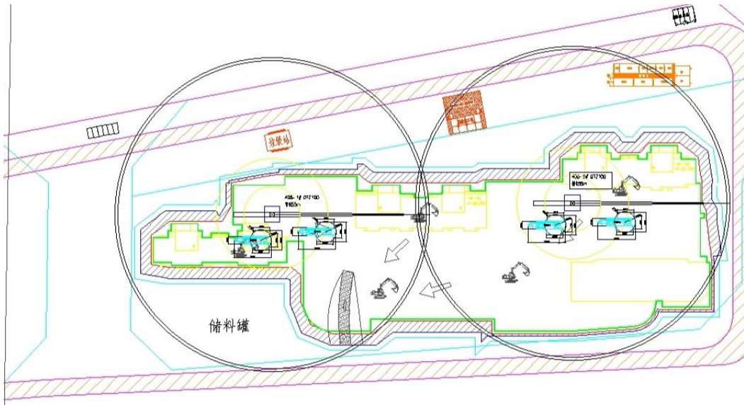
2. 408 地块塔机平面布置图
