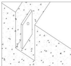
图 3.3-2 接地板图
