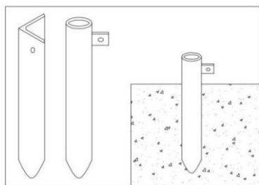
图 3.3-1 接地桩图
