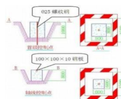
建筑物平面控制网点作法
