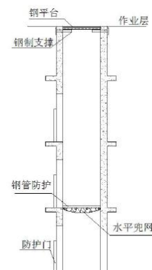
井筒竖向剖面示意图
